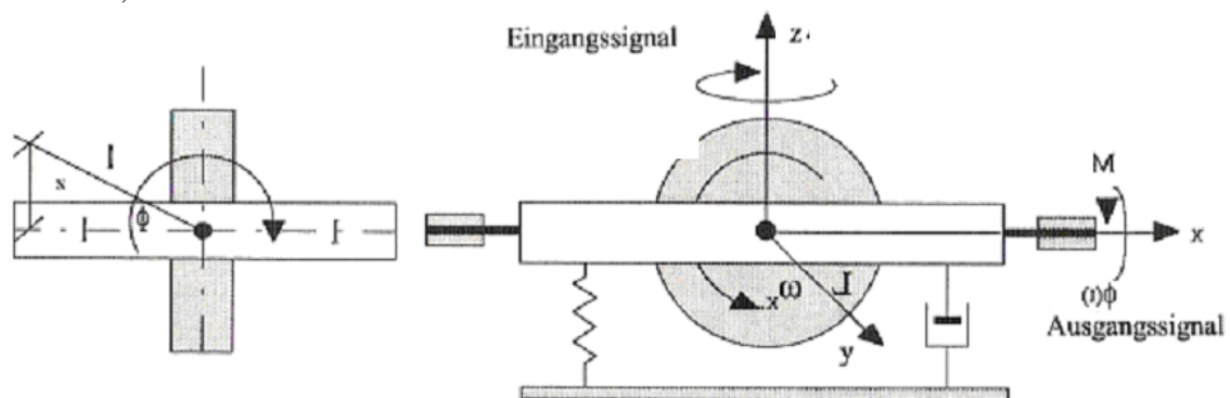
Abb. 9-39 Kennzeichen des Wendekreises ist die Federfesselung des Ausgangs-Rahmens, der proportional zur Winkel-Geschwindigkeit der Eingangsschwerachse (hier z) ausgelenkt wird.
