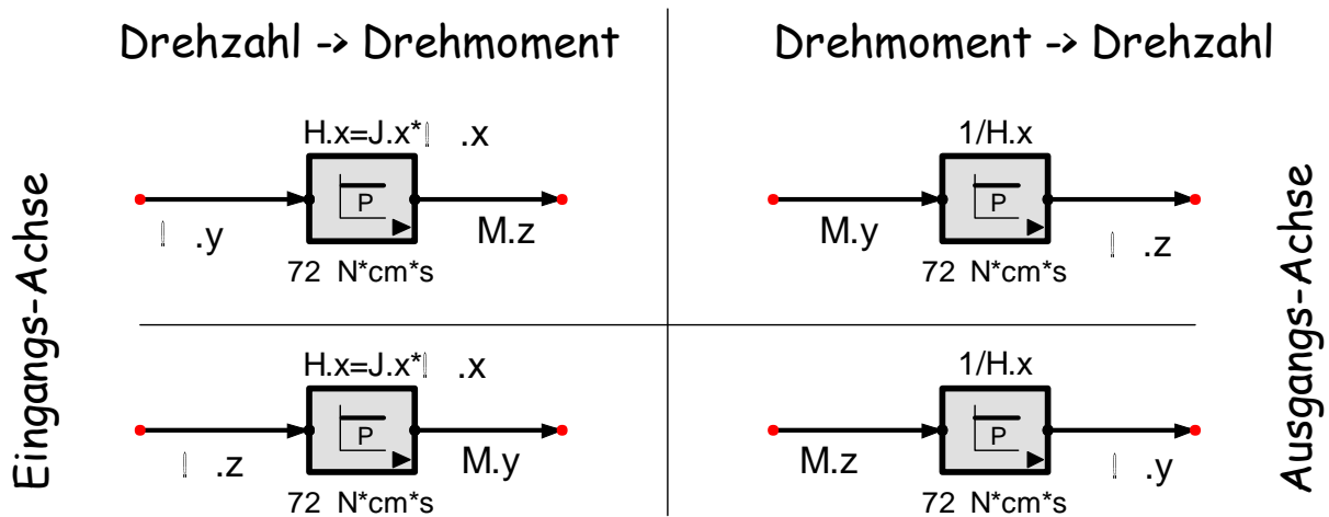
Abb. 9-40 Der Kreisel als Wandler von Drehzahl in Drehmoment und umgekehrt
