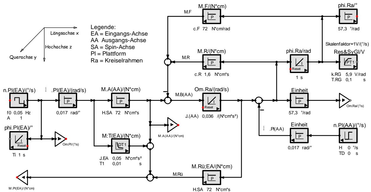
Struktur 9-16 WK-Struktur: Struktur zum Feder-gefederten Kreisels nach Abb. 24. Sie zeigt, wie die Drehungen der Plattform um ihre Querachse y und ihre Hochachse z Auslenkungen um die Querachse y erzeugen.
