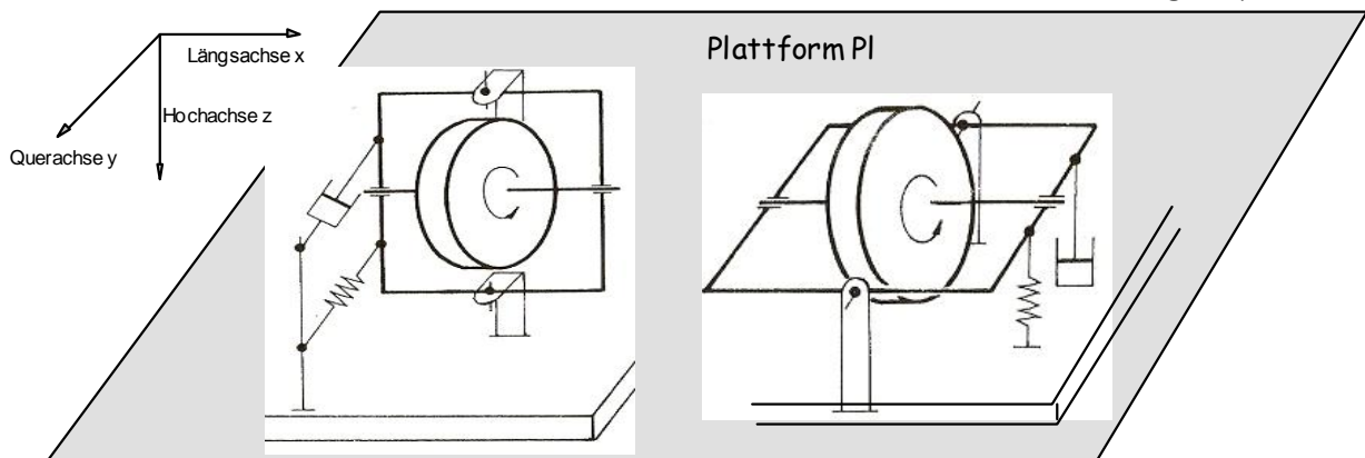
Abb. 9-47 Kreislerplattform zur Messung der inertialen Elevations- und Azimut-Geschwindigkeit.
