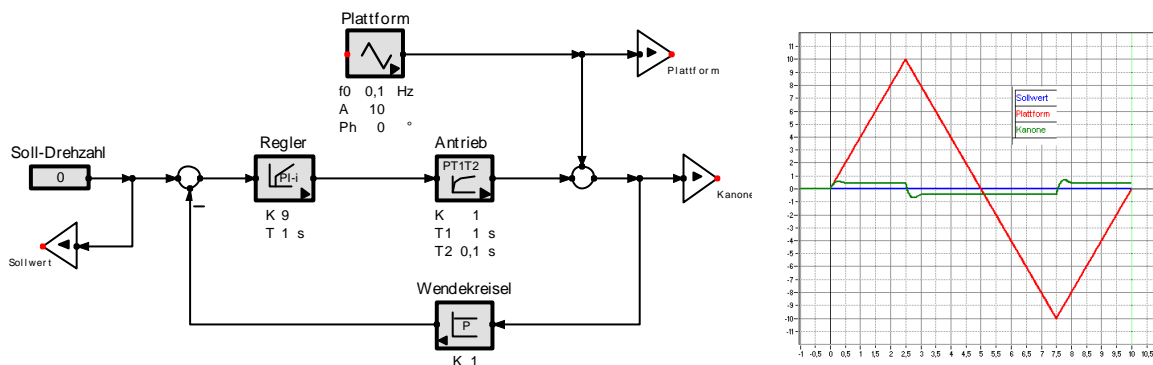
Struktur 9-15 Kanone-Elevation: Regelkreis zur Waffen-Stabilisierung in der Höhe. Vom Richtschützen wird so lange ein Geschwindigkeits-Sollwert vorgegeben, bis die Waffe auf das Ziel zeigt. Danach stabilisiert der Kreis die Lage, so dass aus der Fahrt geschossen werden kann. Als Test wurde eine rampenförmige Bewegung der Plattform (Panzer-Wanne) angenommen. Der Graph zeigt die nicht-ausgeregelter Restgeschwindigkeit der Waffe.
