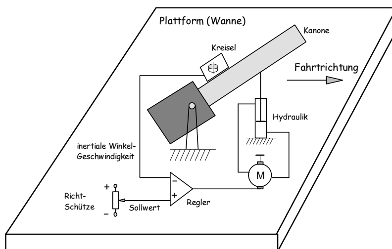
Abb. 9-43 Regelkreis zur Stabilisierung einer Panzer-Kanone in der Höhe (Elevation). Die Kanone soll, nachdem sie auf das Ziel ausgerichtet ist, in Ruhe bleiben, obwohl ihre Aufhängung (die Panzerwanne) sich während der Fahrt dreht. Wenn der Regelkreis funktioniert, stellt der Regler den Hydraulik-Zylinder immer so ein, dass er die Bewegung des Panzers ausgleicht.
