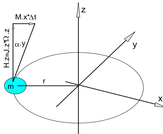
Abb. 9-41 Zur Ableitung der Kreisel-Präzession \Omega.y = H.z \cdot M.x
