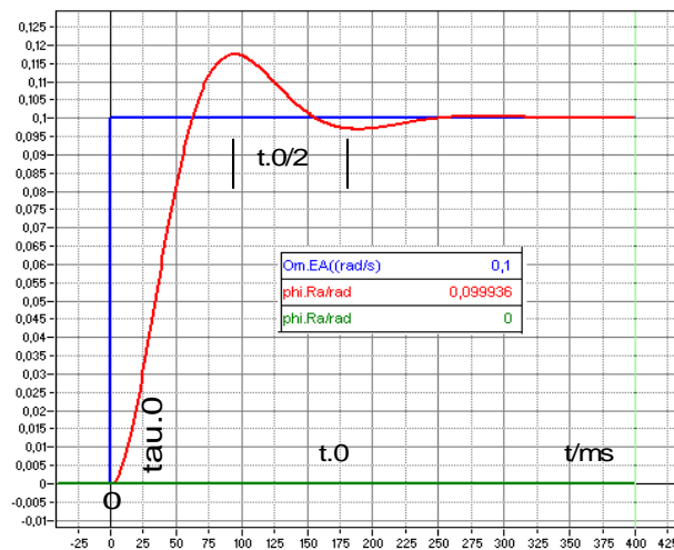
Abb. 9-49 Messung einer inertialen Dreh-Geschwindigkeit durch einen Wende-Kreisel:
