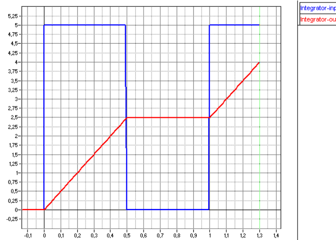
Abb 3-20 Signal- Integration: Integration einer Konstanten
