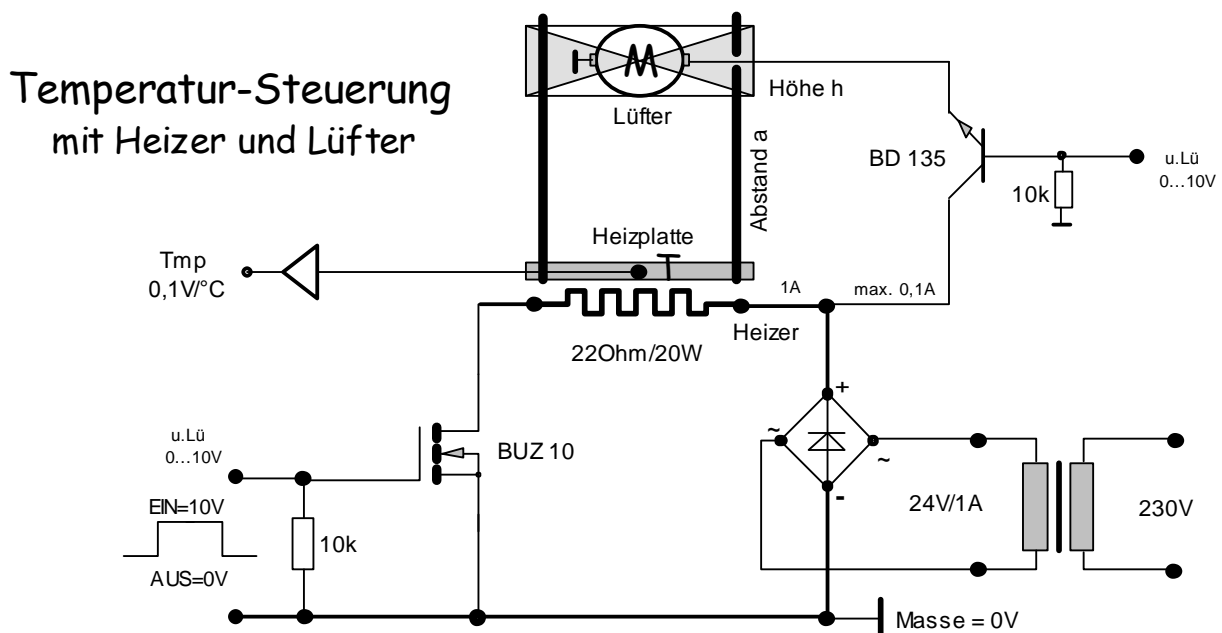
Abb. 13-21 Schema der Heizplatte mit Lüfter. Der Lüfter kann mit Spannungen von 0 bis 12V stetig betrieben werden. Der Heizer sollte für den quasi-stetigen Betrieb über einen Pulsweiten-Modulator angesteuert werden (siehe Kapitel 7 Elektronik\Schaltungstechnik).
