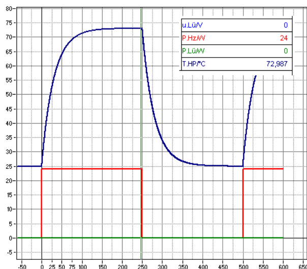
Abb. 13-23 Simulierter Temperaturverlauf bei Heizung ohne Kühlung: Erwärmung und Abkühlung erfolgen mit derselben Zeitkonstanten, hier 30s.
