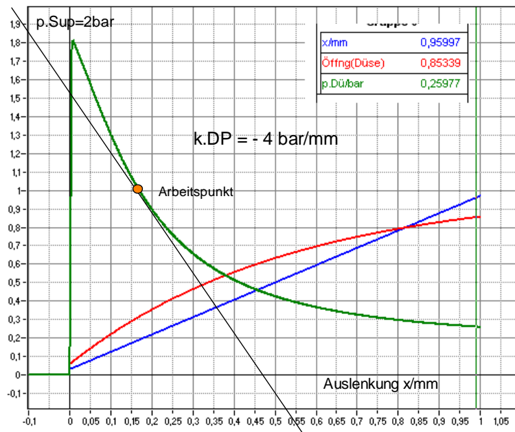
Abb. 12-87 Simulation des Düsendrucks p.Dü bei Variation des Prallplatten-Abstands x. Die Steigung der Tangente im Arbeitspunkt ( p.Dü = p.Sup/2 ) beschreibt die mittlere Empfindlichkeit k.DP des Düse-Prallplatte-Systems. Hier: k.DP = - 4 \text{ bar/mm} .
