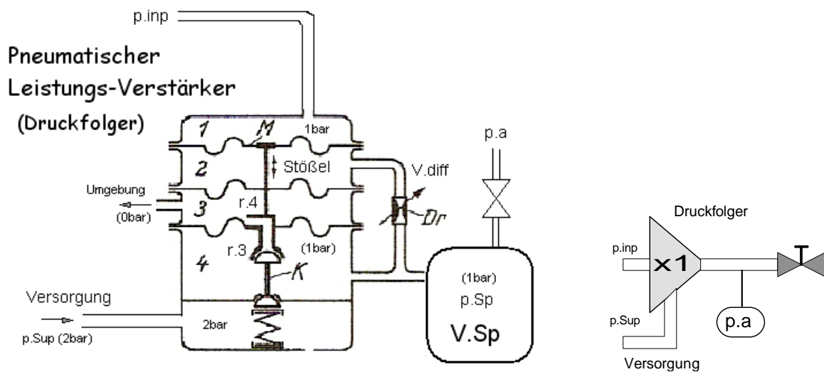
Abb. 12-83 Pneumatischer Leistungs-Verstärker mit 3 Membranen: nicht-blasend. Die Anordnung ist ein Dreipunktregler, der eine Pulsbreiten-Modulation erzeugt: Ist der Speicherdruck p_{.Sp} kleiner als der Eingangsdruck p_{.i} , so wird der Speicher über das Ventil r_{.3} mit der Versorgung verbunden. Der Druck steigt. Ist der Speicherdruck p_{.Sp} größer als der Eingangsdruck p_{.i} , so wird der Speicher über das Ventil r_{.4} mit der Umgebung verbunden. Der Druck sinkt. Stimmt der Speicherdruck mit dem Eingangsdruck p_{.i} überein, so sind beide Ventile geschlossen.
